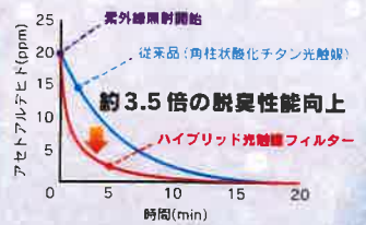
ハイブリッド光触媒は、従来品と比べて約3.5倍の性能向上を達成。
